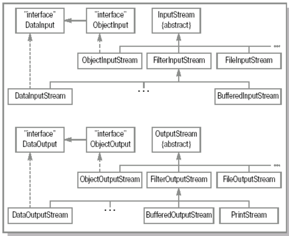
Рис. 1. Иерархия классов ввода/вывода.
