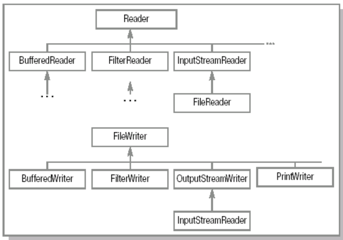
Рис. 2. Иерархия классов Reader и Writer.
