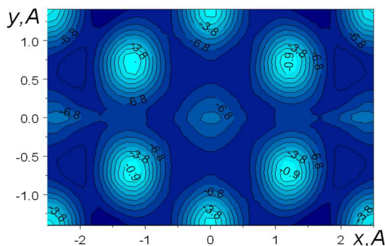
Рис. Проекція потенціальної енергії взаємодії вуглецевого пробника з графеном
