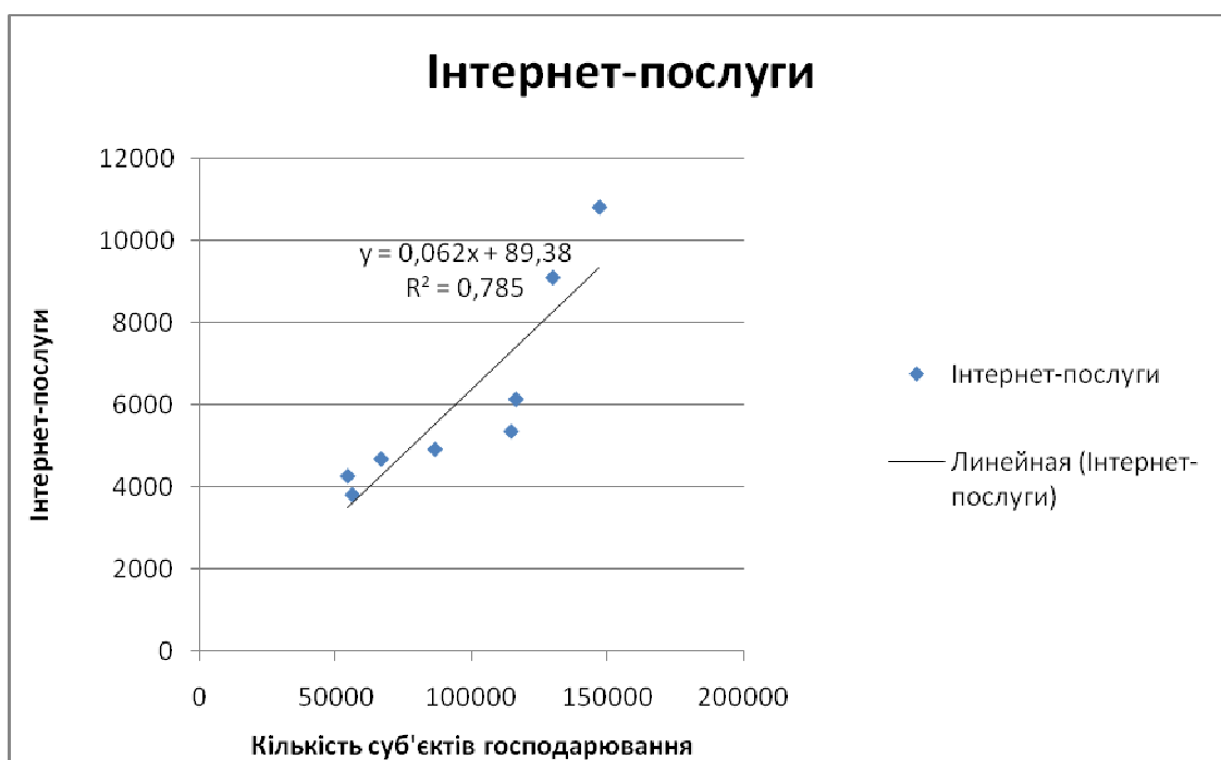
Рис. 2. Поле кореляції між інтернет-послугами та кількістю суб'єктів господарювання у сфері інформації й телекомунікації
